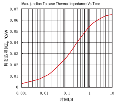
Fig.2 结至管壳瞬态热阻抗曲线
