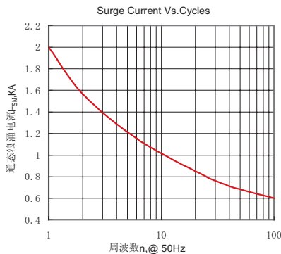
Fig.7 通态浪涌电流与周波数的关系曲线
