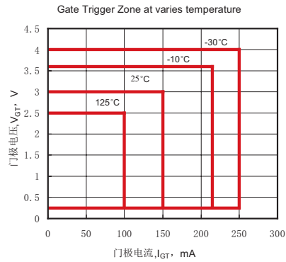
Fig.10 门极触发特性曲线
