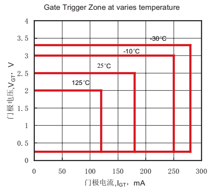
Fig.6 门极触发特性曲线
