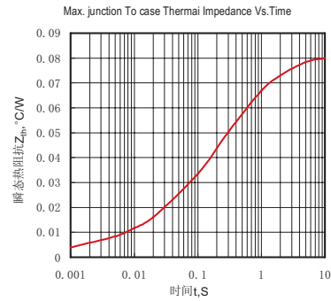
Fig.2 结至管壳瞬态热阻曲线
