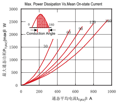
Fig.3 最大功耗与平均电流关系曲线
