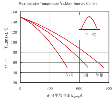
Fig.4散热器温度正向平均电流 关系曲线
