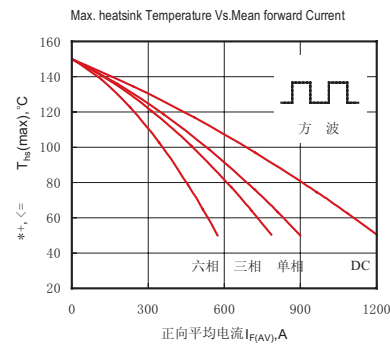
Fig.6 散热器温度正向平均电流 关系曲线
