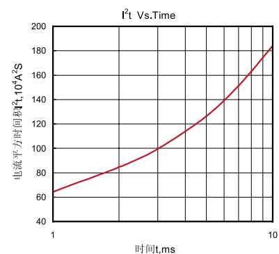
Fig.8 I²t特性曲线
