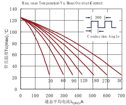
Fig.6 管壳温度与通态平均电流关系曲线
