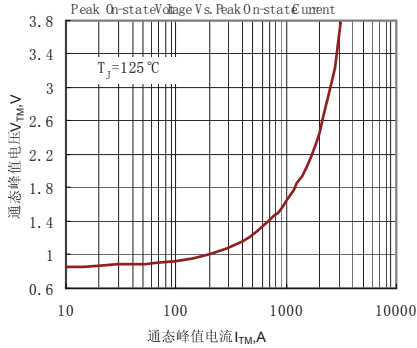
Fig.1 通态伏安特性曲线
