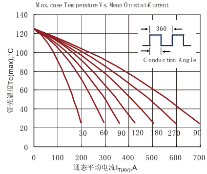
Fig.6 管壳温度与通态平均电流关系曲线
