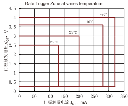
Fig.10 门极触发特性曲线
