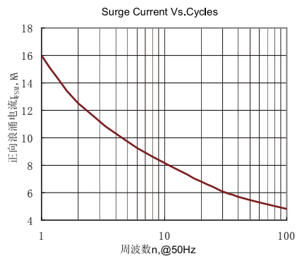
Fig.7 正向浪涌电流与周波数的关系曲线
