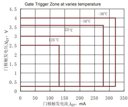
Fig.10 门极触发特性曲线
